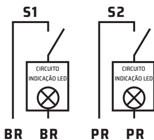
Ligação elétrica
