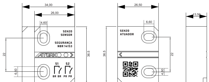
Desenho técnico, sem escala
